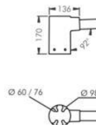
STOLPTOPPSFÄSTE
