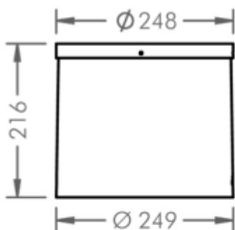
Flushat montage
