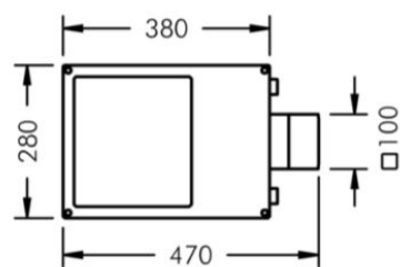
VÄGGFÄSTE
