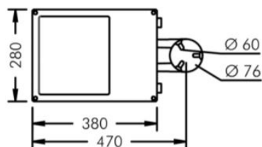
STOLPFÄSTE SINGEL
