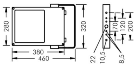
BYGEL
