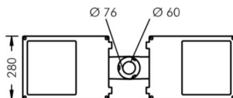
STOLPFÄSTE DUBBEL
