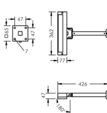
VÄGGARM
