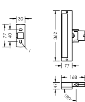
SKENA/ FLÄNS
