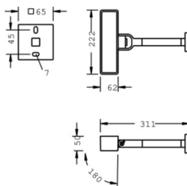
VÄGGARM
