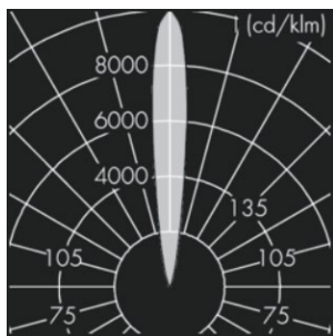
SMALSTRÅLANDE
