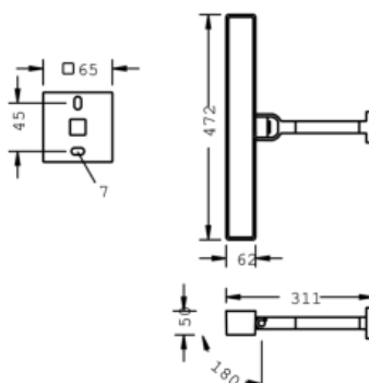
VÄGGARM
