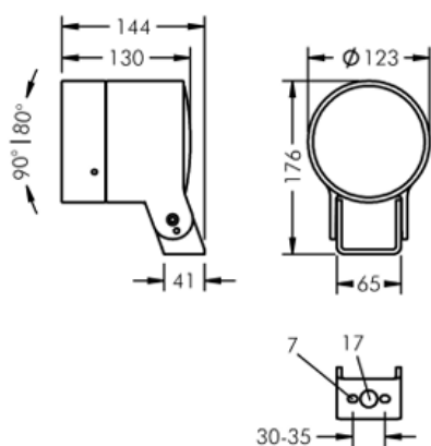
BYGELFÄSTE
