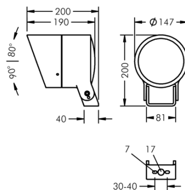
BYGELFÄSTE + KEPS
