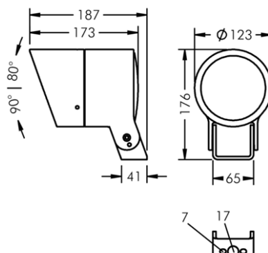
BYGELFÄSTE + KEPS
