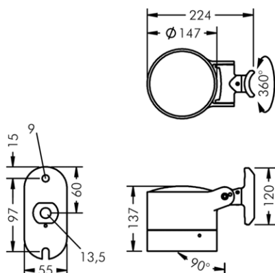
STOLPFÄSTE Ø 60-100mm
