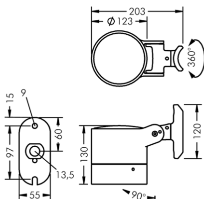
STOLPFÄSTE Ø 60-100mm
