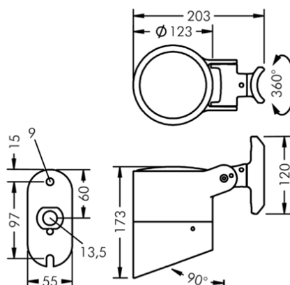
STOLPFÄSTE + KEPS
